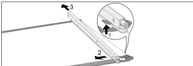
Fig. 84 Üveglap sínekkal
