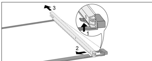
Fig. 82 Üveglap sínekkel
