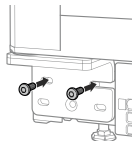
22. Csavarozza fel a csuklópántot.
