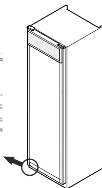
21. Fordítsa el jobbra a zsanéridomot. A zárószervezetben lévő rugó ezzel megfeszül.
