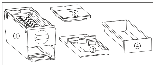
Fig. 93 Az EasyTwist-Ice alkotórészei
